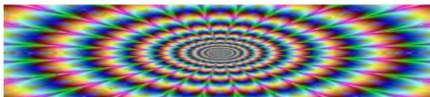
Figura 37 - Esperienza psichedelica indotta da LSD
