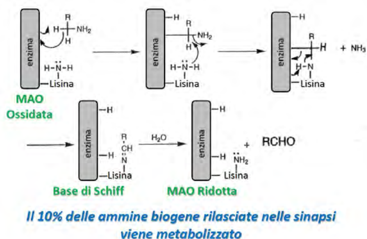
Figura 17 - MAO: meccanismo di ossidazione
