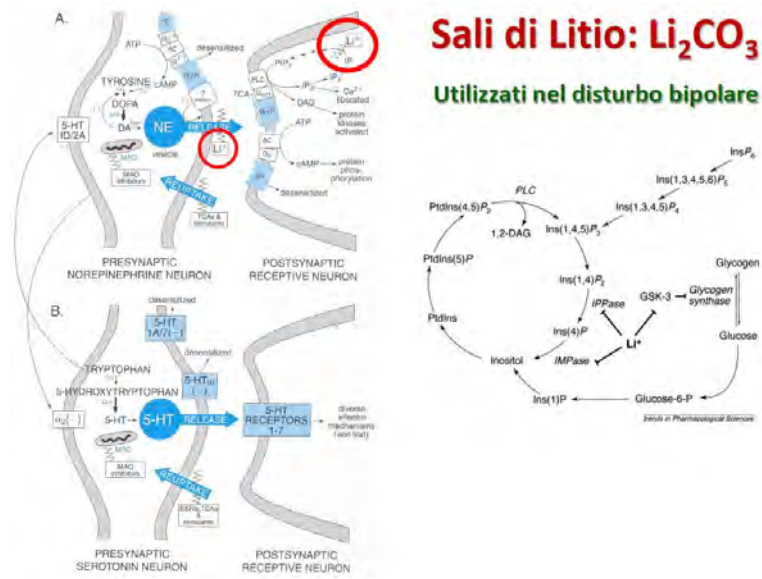
Figura 56 - Sali di litio: \text{Li}_2\text{CO}_3 utilizzati nel disturbo bipolare
