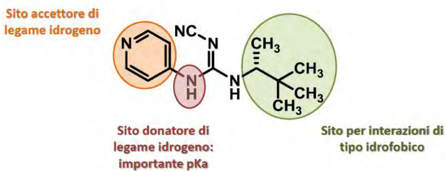
Figura 38 - Cianoguanidine: Pinacidil
