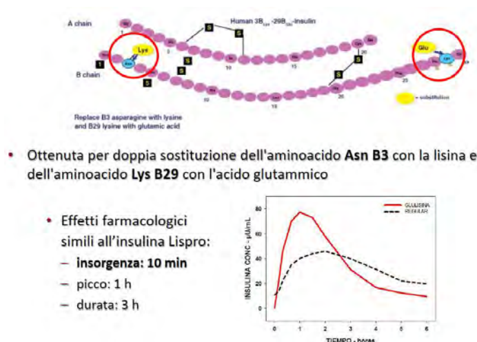
Figura 43 - Insuline ultrarapide: Glulisina - Aprida
