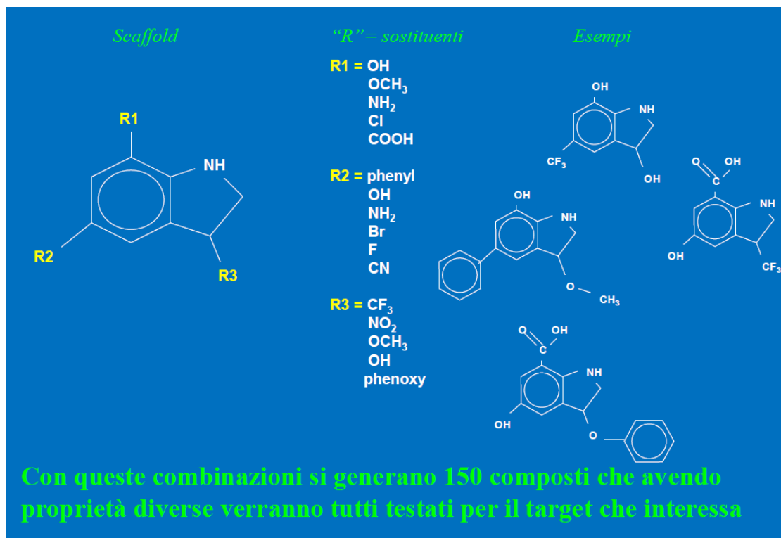
Figura 10 - Chimica Combinatoria
