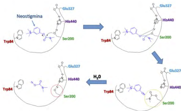
Figura 25 - Meccanismo di carbamilaione AChE
