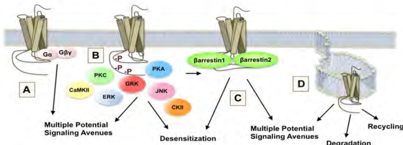
Figura 33 - Morfina e \beta -arrestina
